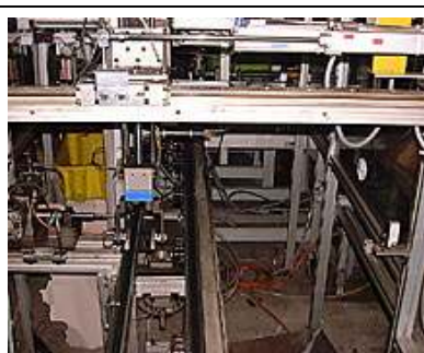
Vollautomatische Montageeinrichtung für Schwerlast Rollen 300 Kg Traglast (Abb. 2)
